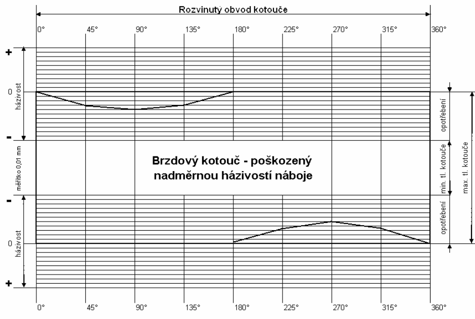
Graf házivosti a opotřebení brzdového kotouče
